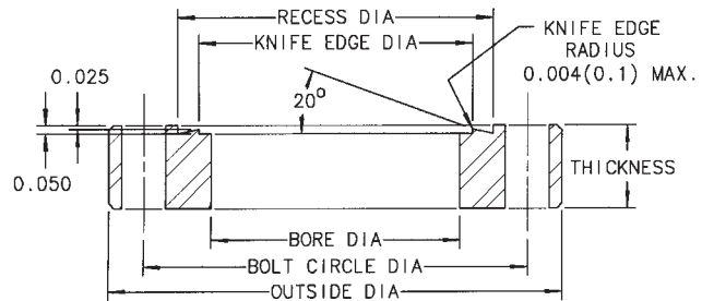
Flange Multiplexer MCF275-FM4R04-A
